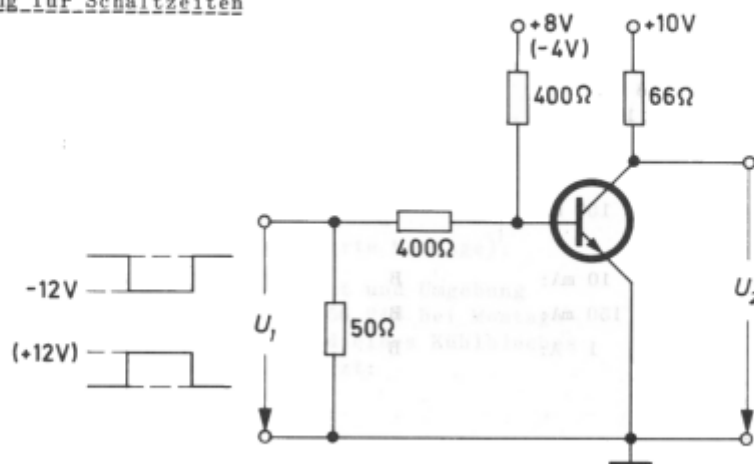
Schaltzeit-Messung mit Zweistrahl-Oszillograf ( t_r \leq 5\text{ ns} )
